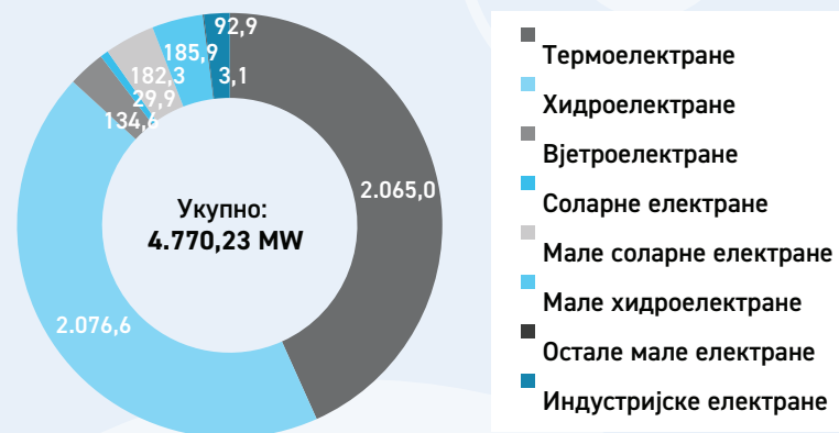
Инсталирана снага производних објеката у Босни и Херцеговини, 31. децембра 2023. (MW)
